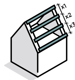
MEERVELDS OVERSPANNING
