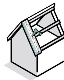
BEVESTIGING DWARSE OVERSTEEK
